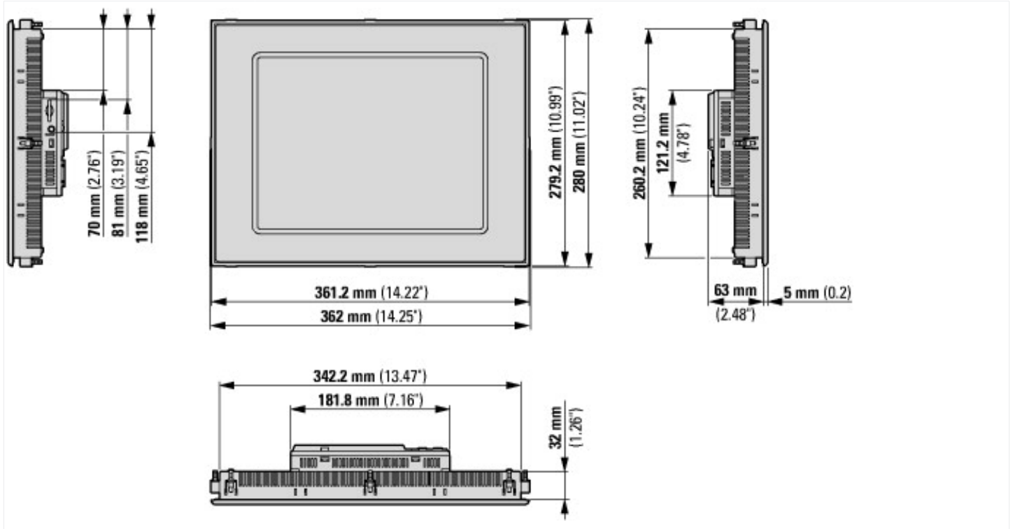
Écran tactile XV-363... version écran avec diagonale de 12,1 pouces : Montage encastré
