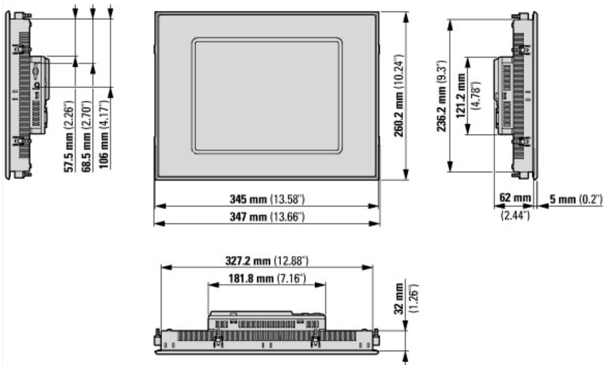
XV-363-berøringspanel ... versjon med 10,4-tommers diagonal skjerm: Planmontering
