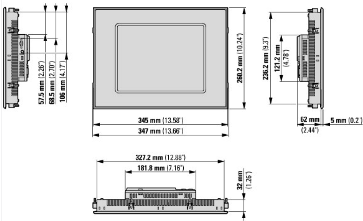
Écran tactile XV-363... version écran avec diagonale de 10,4 pouces : Montage encastré
