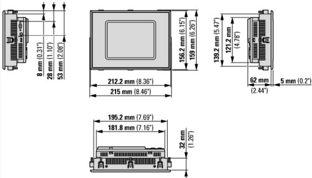
XV-363-... touchpaneel versie met 5,7-inch beeldscherm diagonaal: Installatie
