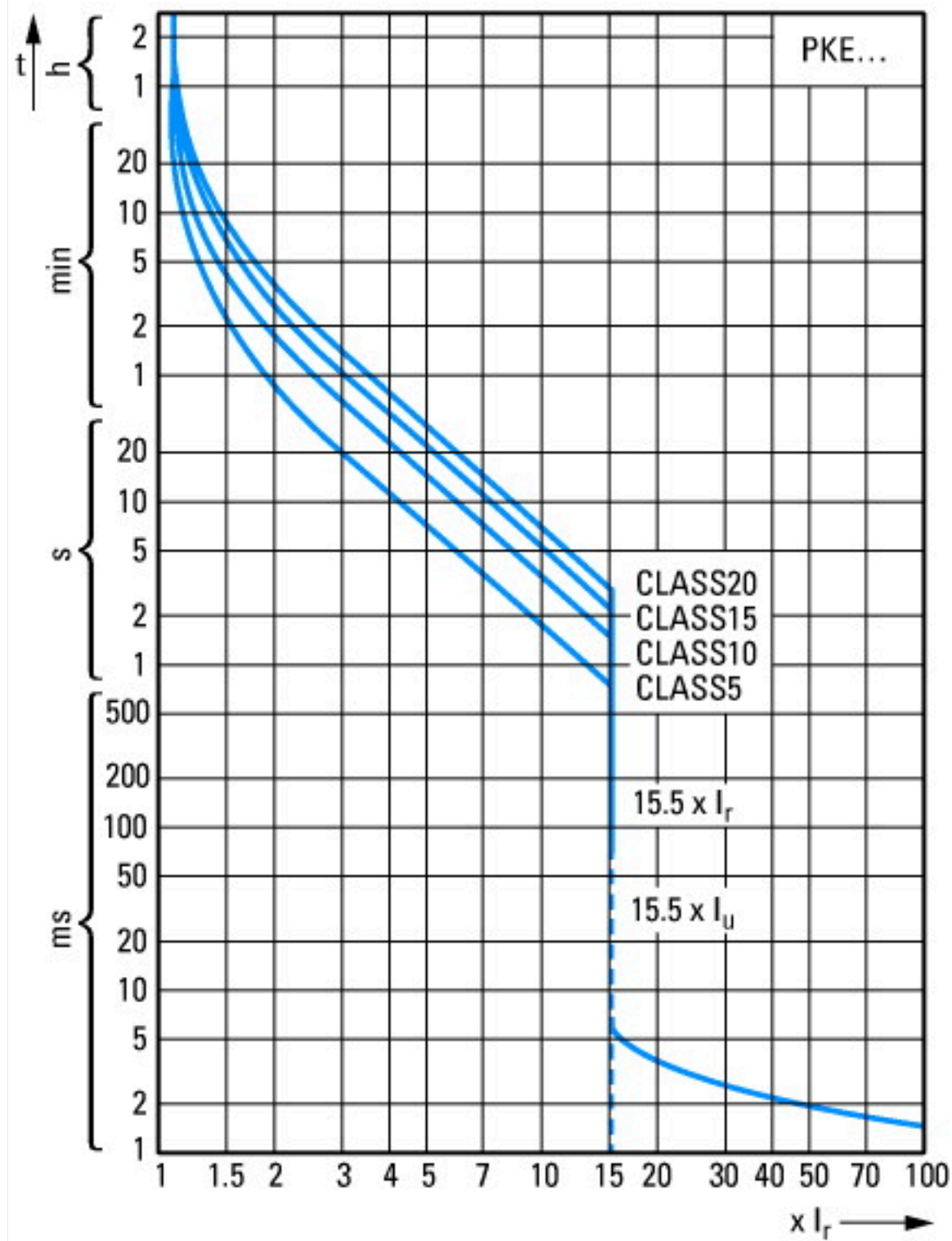
Auslösekennlinien
