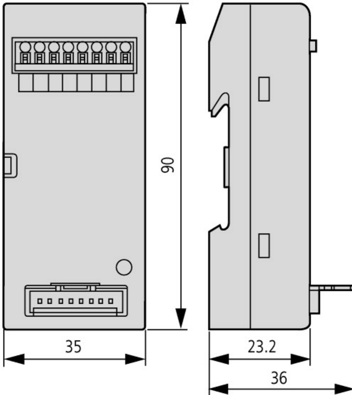
Adapter vlakbandkabel (stekker) naar rondkabel (klem)
