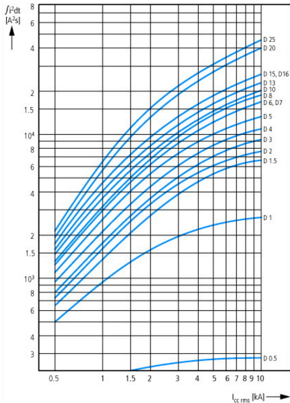
Contrainte thermique I^2t Caractéristique D (0,5 - 20 A), 277 V
