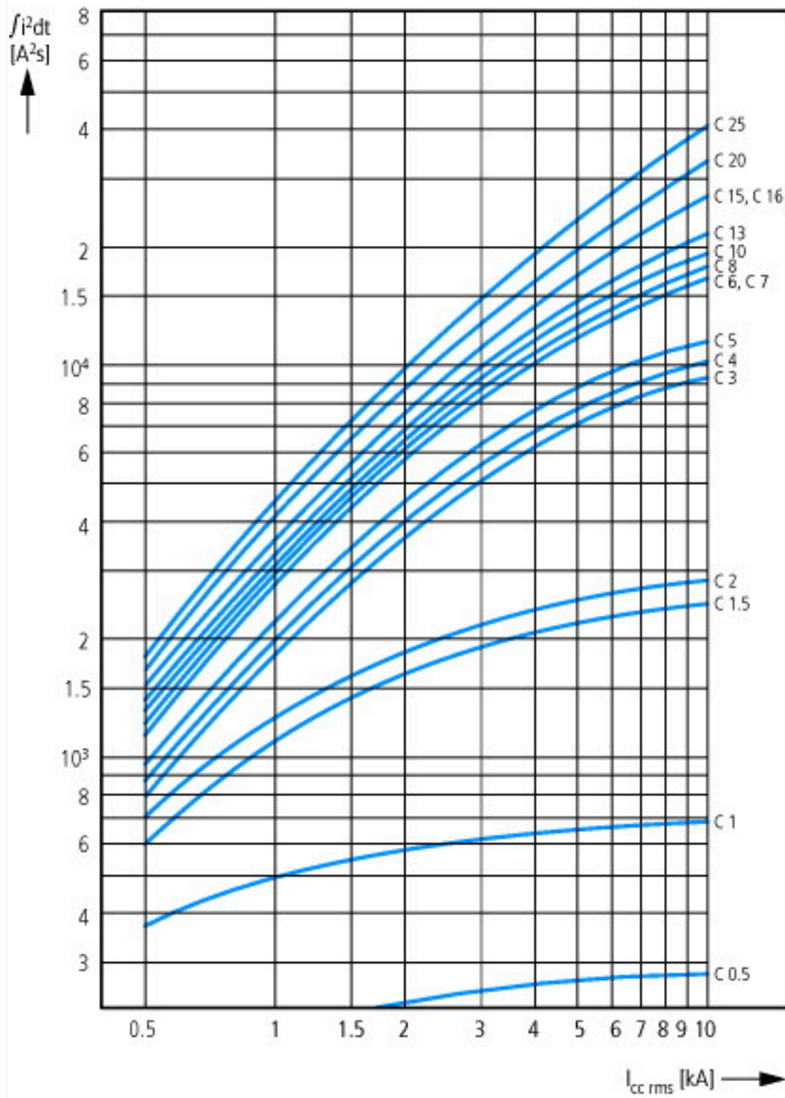
Doorlaatenergie i^2t Karakteristiek C (0,5 - 20 A), 277 V
